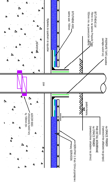
Typowy przekrój stropu / tarasu z wykończeniem PRZEKRÓJ
